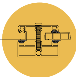
Bevestiging van polycarbonaat in een zijsluitprofiel.
